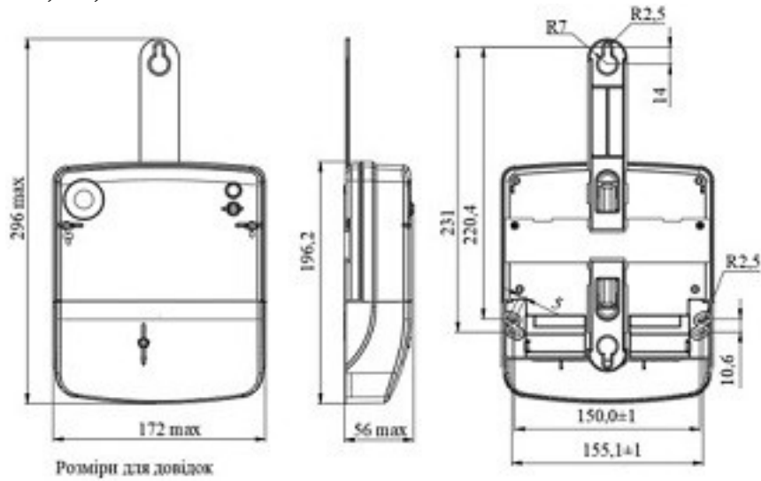
Рисунок 1. Габаритні та установочні розміри лічильника
